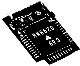
■ CTCSS UNIT TSU-6
