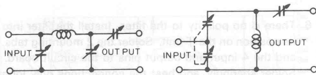
Fig. 5-10 Matching Circuits
